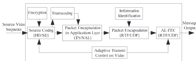
Fig. 3. Aspecto técnico del proveedor, gentileza de [2]
