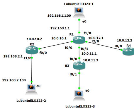
Fig. 6. Topología de red a simular
