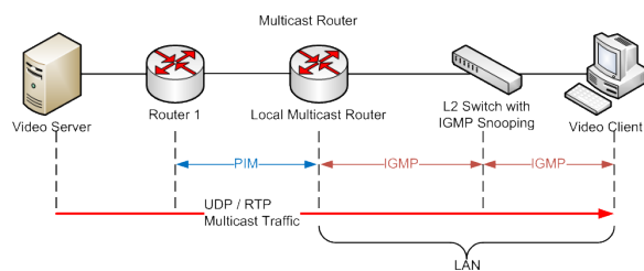
Fig. 5. Arquitectura de transmisión multicast
