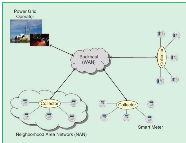
Figura 1. Estructura de red AMI. [3]
