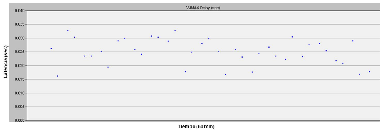
Figura 10. Latencia en los enlaces WiMAX
