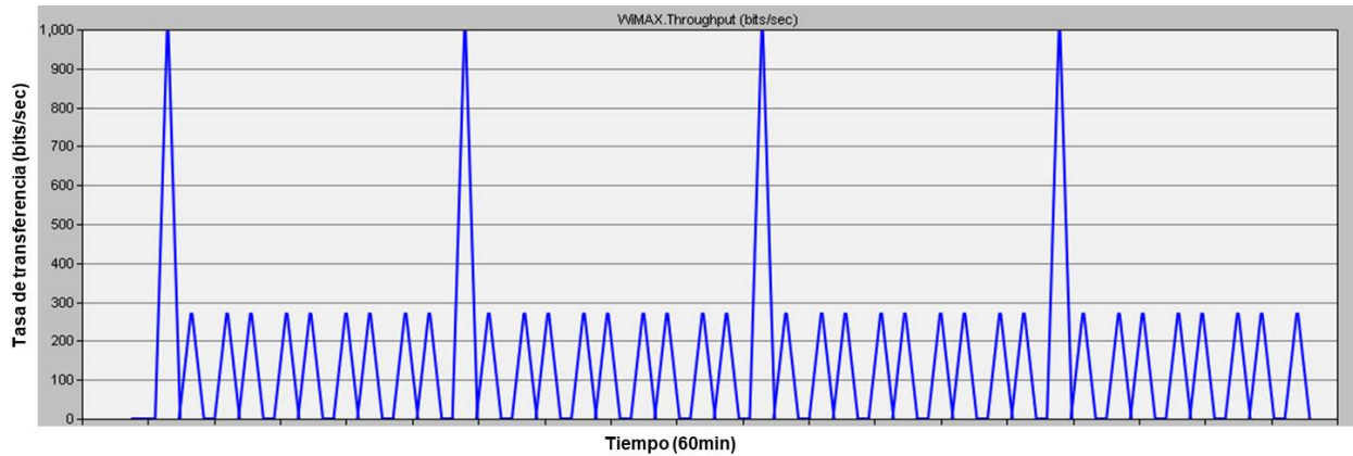
Figura 9. Tasa de transferencia en los enlaces Wimax
