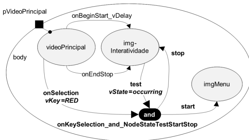
Figura 10.16 Visão estrutural com elo que utiliza um conector com condição composta.
