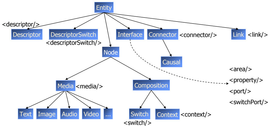
Figura 2.5 Entidades NCM e elementos da linguagem NCL.
