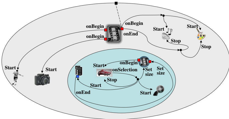
Figura G.2 Visão estrutural da aplicação O Primeiro João .
