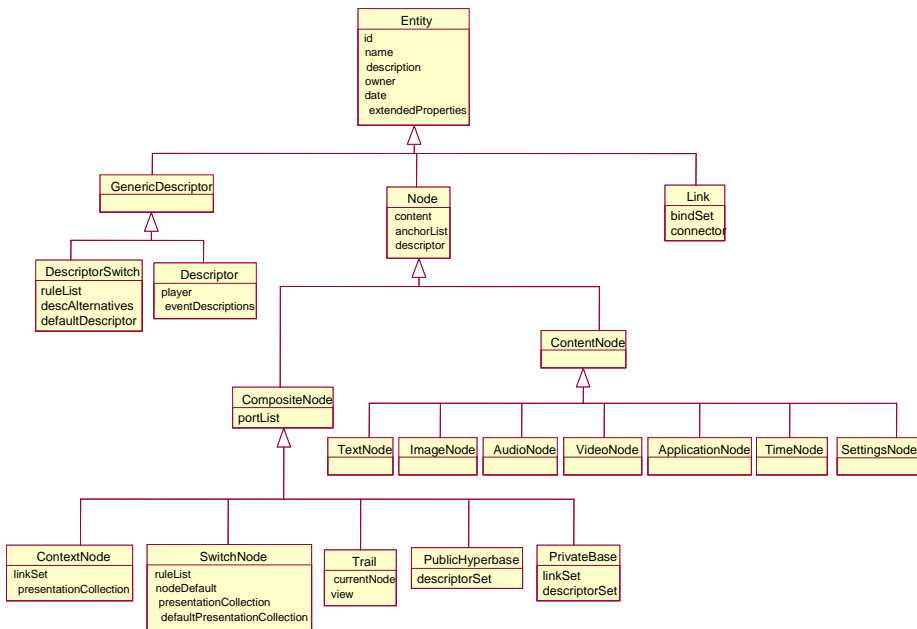
Figura C.1 Visão geral da hierarquia de classes do NCM. 4
