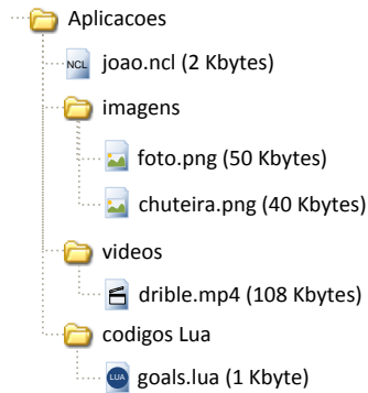
Figura B.3 Árvore de diretórios para um carrossel.
