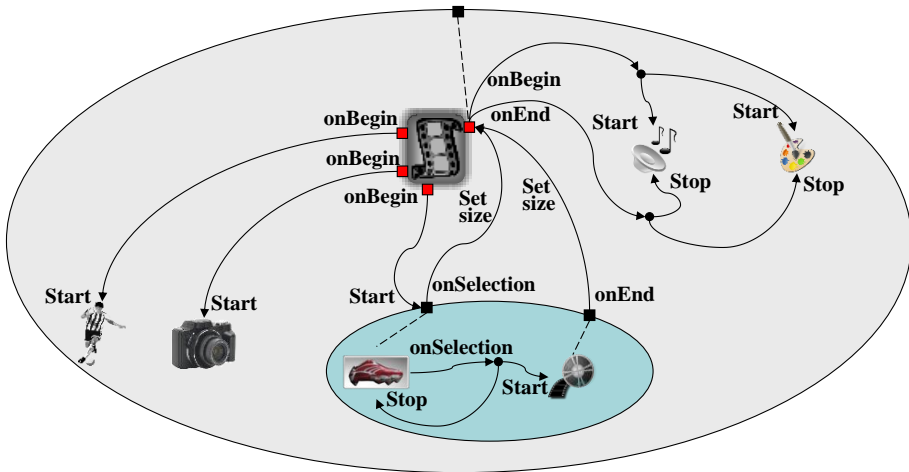
Figura 3.7 Cenas da aplicação O Primeiro João usando contextos.
