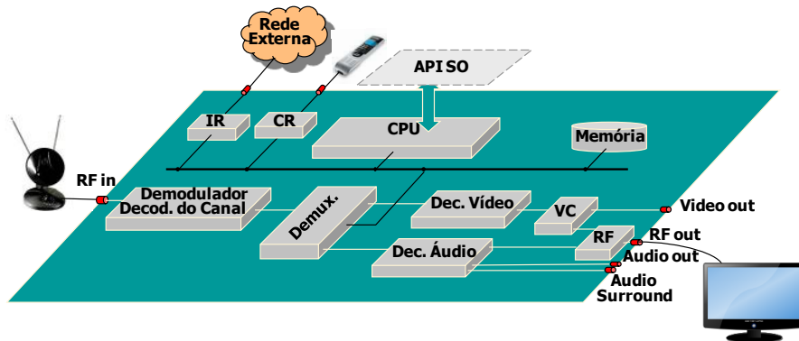
Figura 1.3 Receptor de TV digital.
