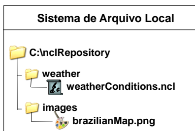
Figura 16.1 Sistema de arquivos do documento a ser adicionado.
