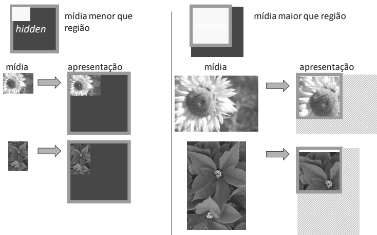
Figura 7.6 Ilustração do parâmetro de descritor fit com o valor “hidden”.
