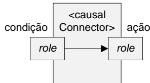
Figura 10.1 Ilustração de um conector causal (elemento <causalConnector> ) com papéis ( role ) de condição e ação.
