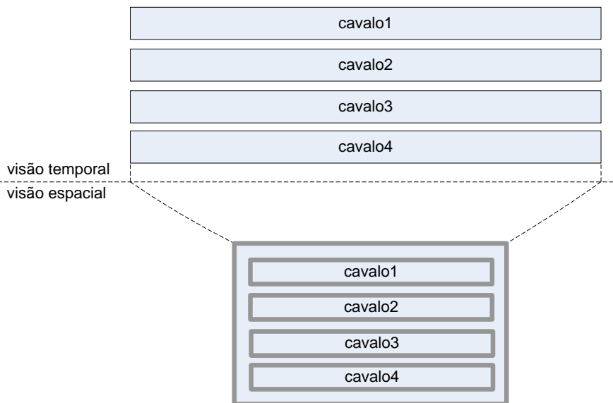
Figura 18.11 Visões temporal e espacial do Exemplo 18.5.
